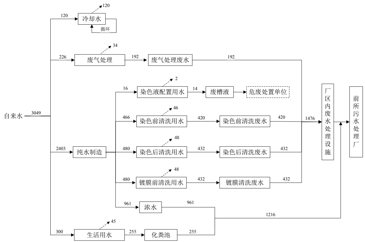
图 5-3 本项目全厂用水平衡图
