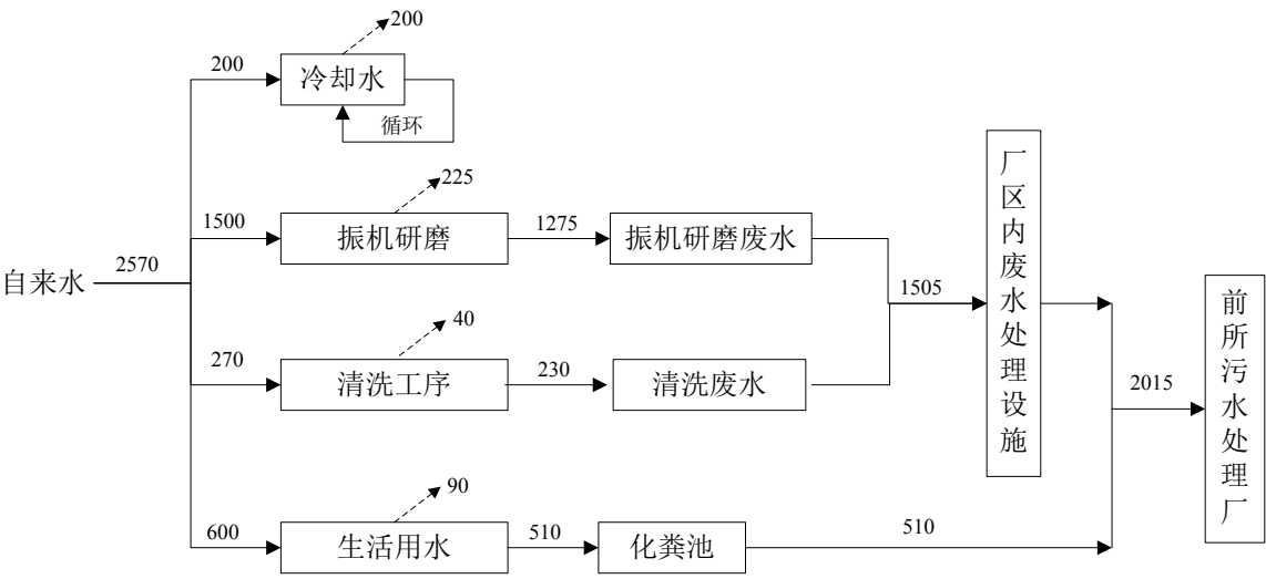
图 5-2 本项目全厂用水平衡图
